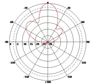
2.4 GHz: E-Plane
