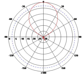
2.4 GHz: E-Plane
