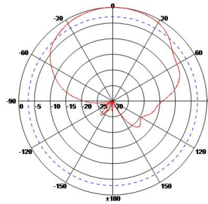
2.4 GHz: H-Plane
